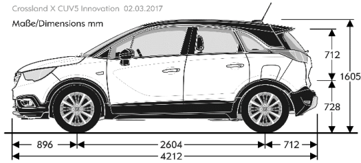
Maße/Dimensions mm
